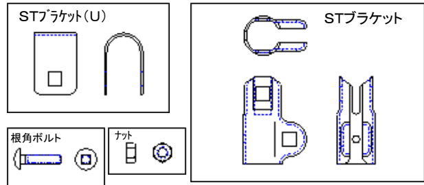
STブラケット Lタイプ 規格表
